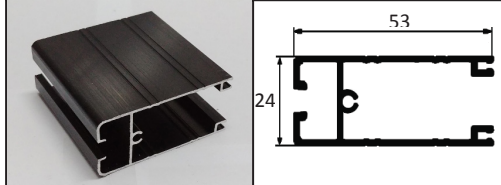
GM-99911 TRANSOM HEADER
