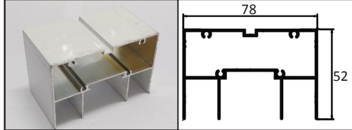
GM-99917 TRANSOM SILL
