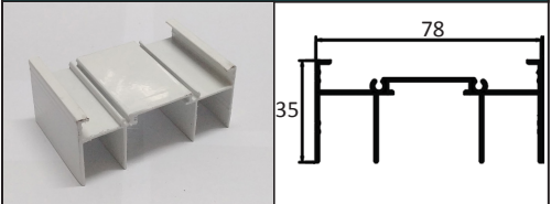
GM-99903 DOUBLE JAMB
