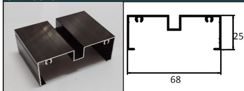
GM-79812 JAMB MOULDING
